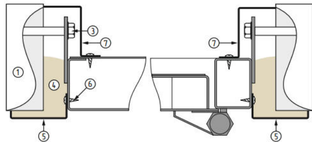
Пример монтажа наличников Вид сверху
