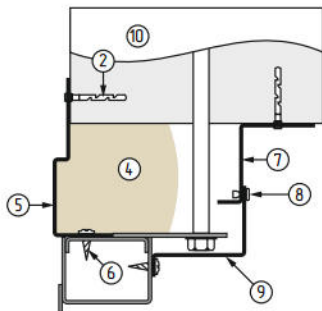
Пример монтажа наличников Вид сбоку
