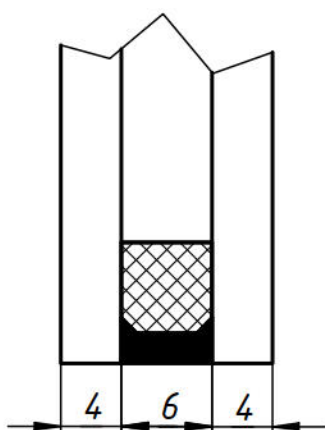
стеклопакет 4-6-4И, 150x1000 мм., один/два, бронзовое тонирование 60%
