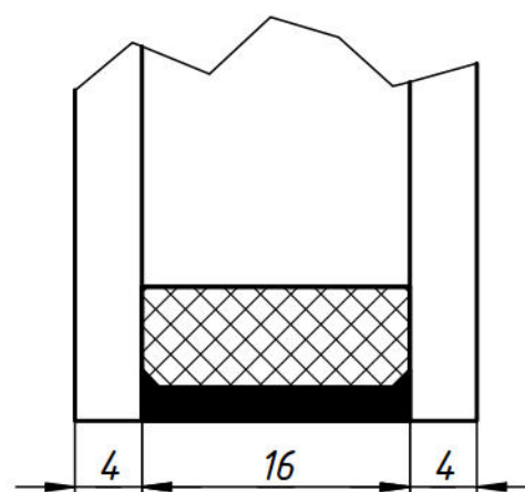
стеклопакет 4-16-4И, 330x1500 мм., один, серое тонирование 60%
