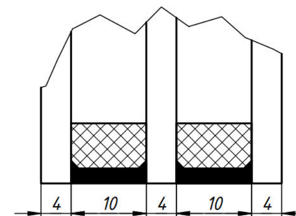
стеклопакет 4-10-4-10-4И, 330x1500 мм., один, серое тонирование 60%
